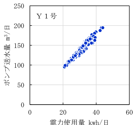
図 2.4 電力使用量とポンプ送水量の関係 (Y 1 号 2021 年度)
