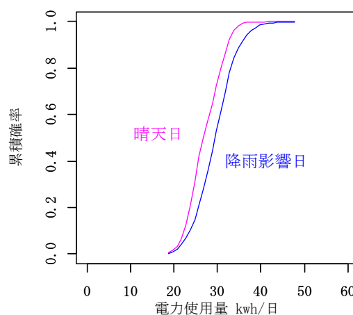
図 3.2 晴天日と降雨影響日の電力使用量の累積確率 (Y 1 号)
