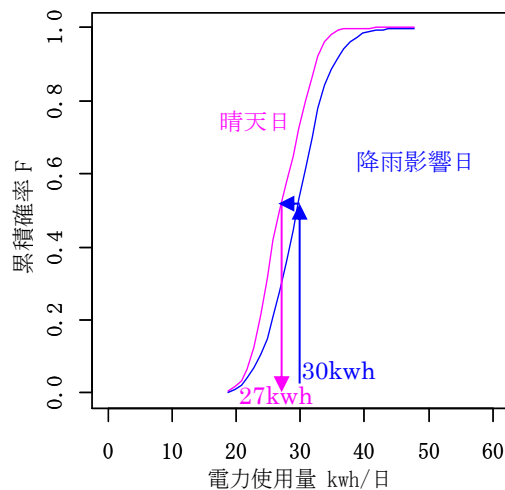
図 3.3 累積確率を使った降雨影響日の降雨の影響の無い電力使用量の推定 (Y 1 号)
