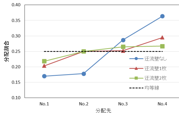
図-6 迂流壁による分配割合の改善挙動
