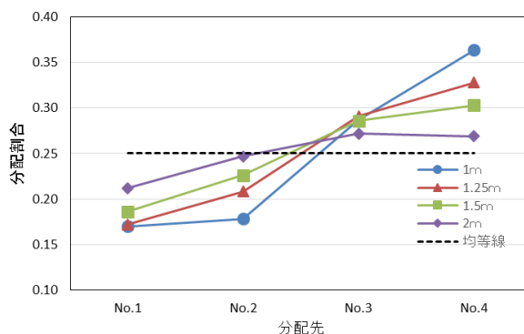
図-5 水路幅により流速を変化させた場合の分配割合の挙動
