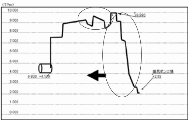
図- 2 圧送管部高低差関係図
