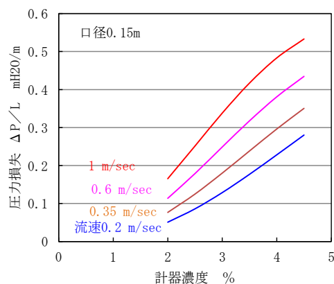
図 4.1 口径 150mm の管内流速別、計器濃度 C と圧力損失 (ΔP/L)
