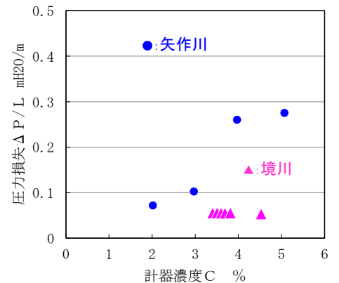
図 3.2 平均計器濃度と平均差圧の関係
