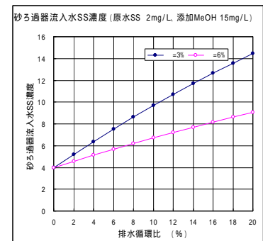
図 - 5 排水循環比と流入 SS 濃度
