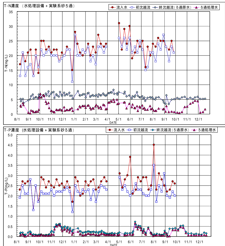
図 - 2 各工程における T-N, T-P 濃度
