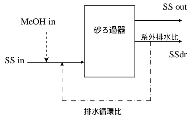
図 - 4 砂ろ過システムの SS 収支図
