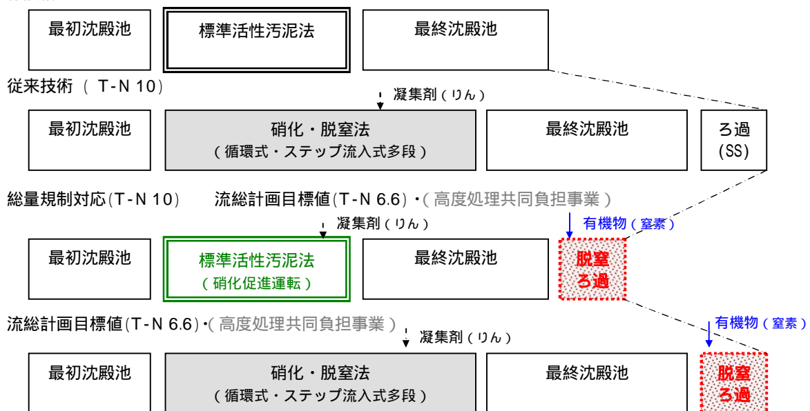
図 - 1 高度処理システムのフロー
