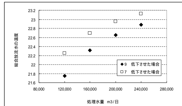
図3 処理水量vs安定化池の放熱効果
