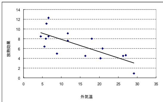
図2 外気温vs安定化池の放熱効果
